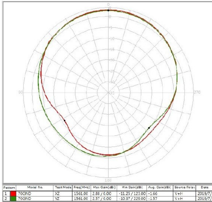
XZ+YZ -Plane 1561 MHz
