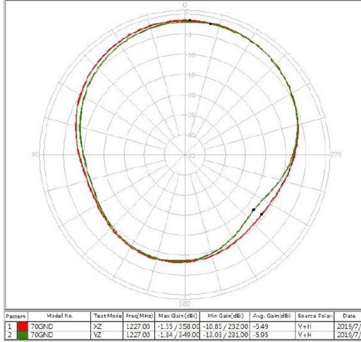
XZ+YZ -Plane 1227 MHz
