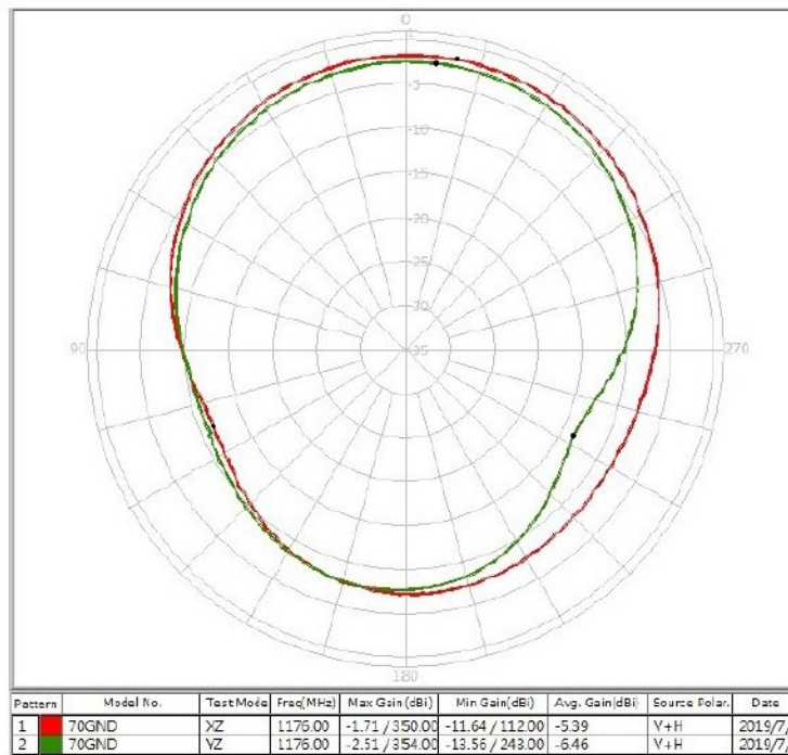
XZ+YZ -Plane 1176 MHz
