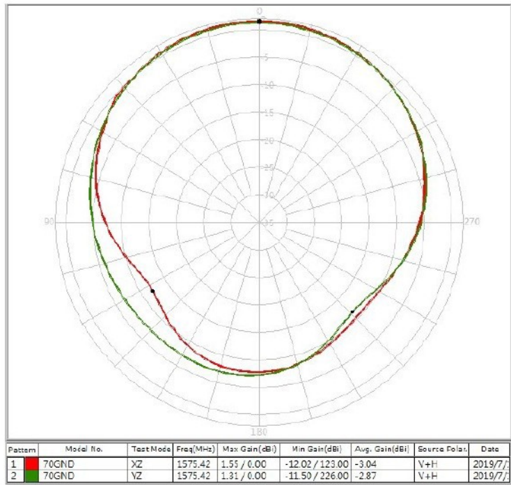
XZ+YZ -Plane 1575.42 MHz
