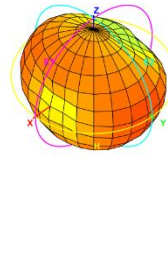
Total_3D_Front View_960MHz
