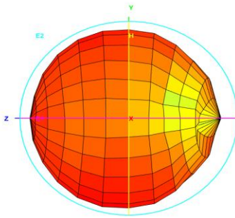
Total_3D_Top View_1.8GHz
